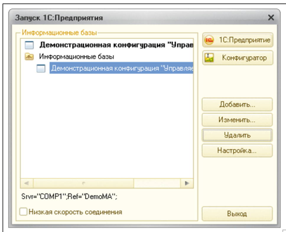
Рисунок 17. Запуск «1С:Предприятия»
