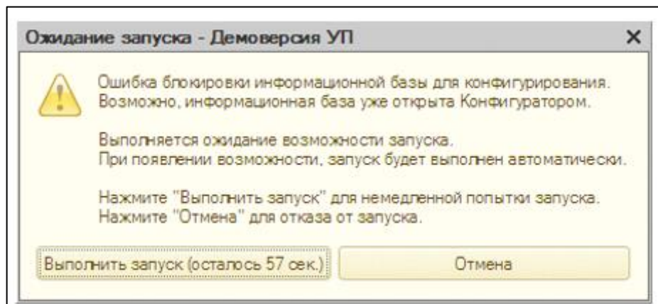
Рисунок 19. Ожидание перезапуска
