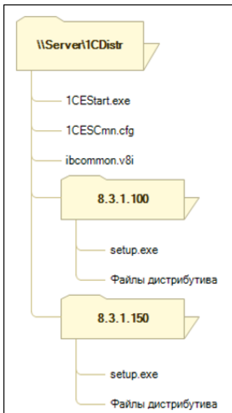
Рисунок 10. Структура каталога
