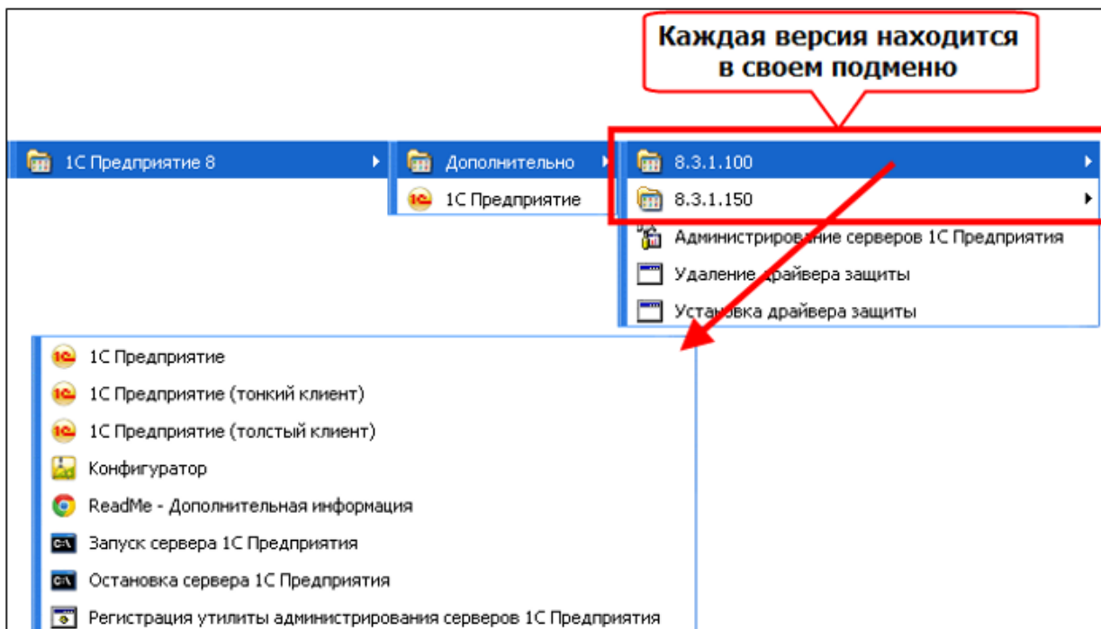
Рисунок 15. Структура меню
